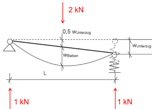
Abbildung 5: Rechenmodell für nachgiebig gelagerte Decken
